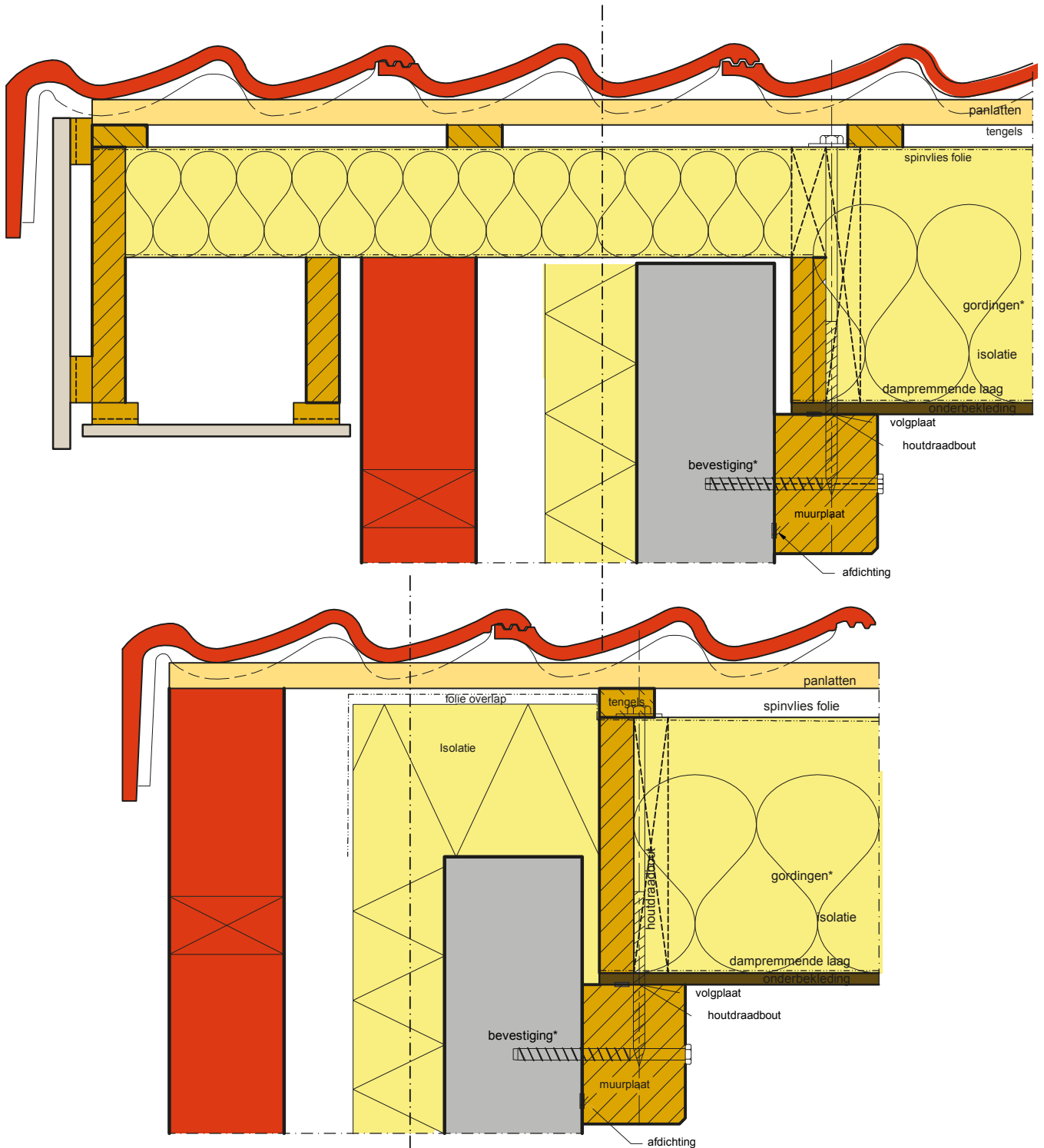
Detail 25: dakoverstekconstructie (gording)
