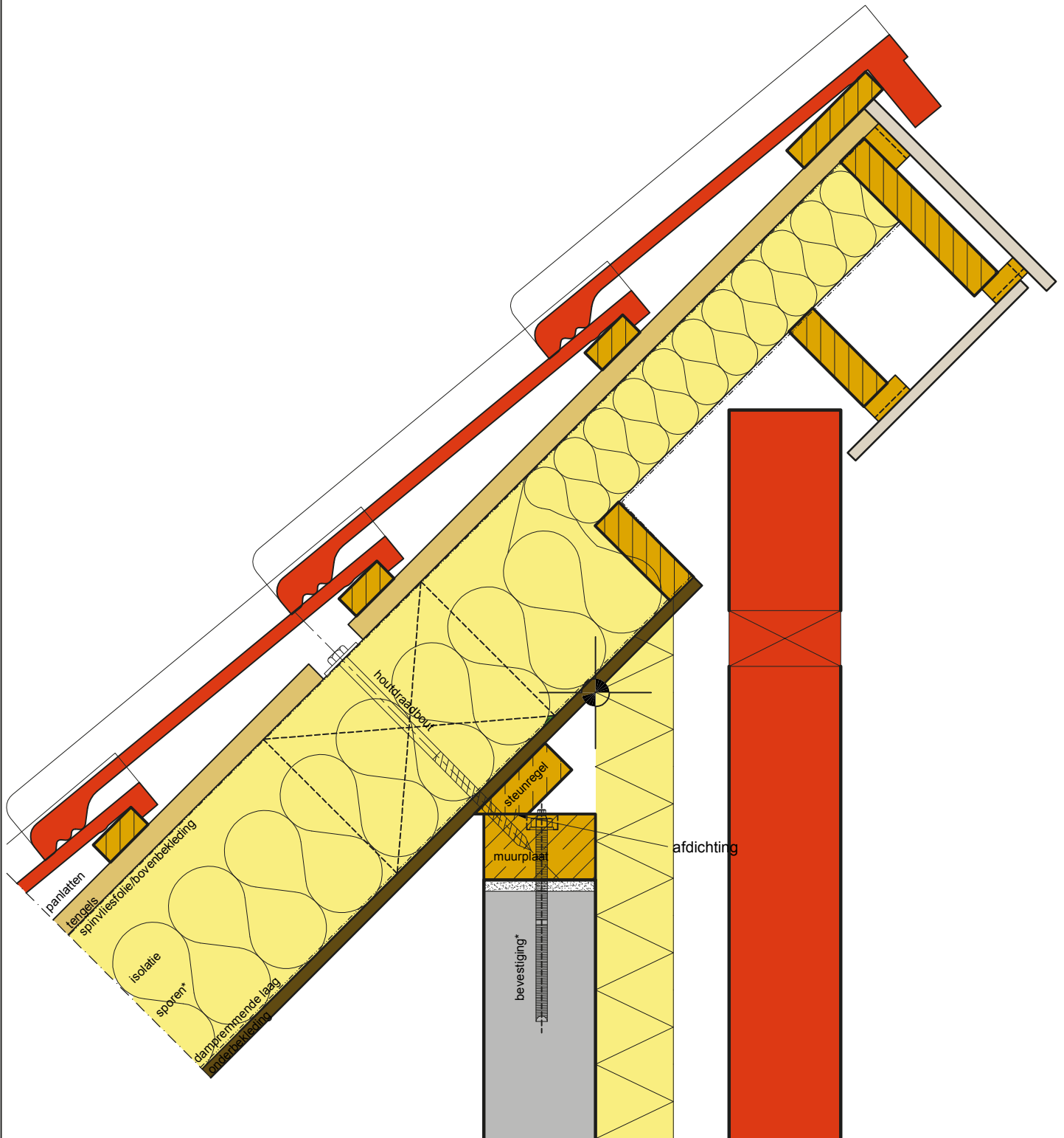
Detail 9: nok lessenaarsdakconstructie
