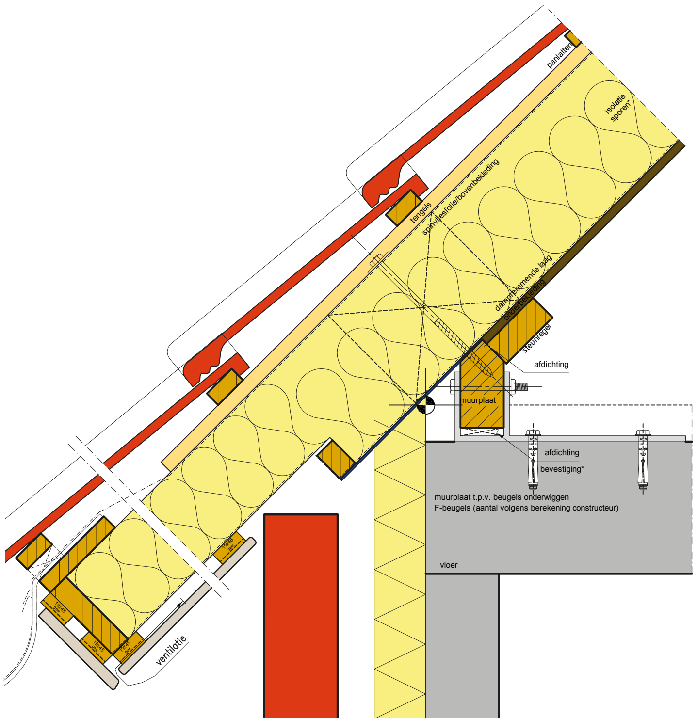
Detail 18: dakoverstekconstructie
