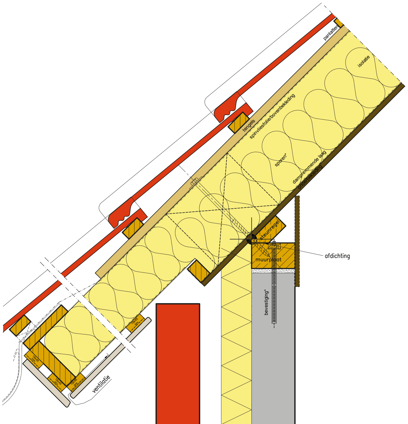
Detail 10: aansluiting borstwering-dakconstructie
