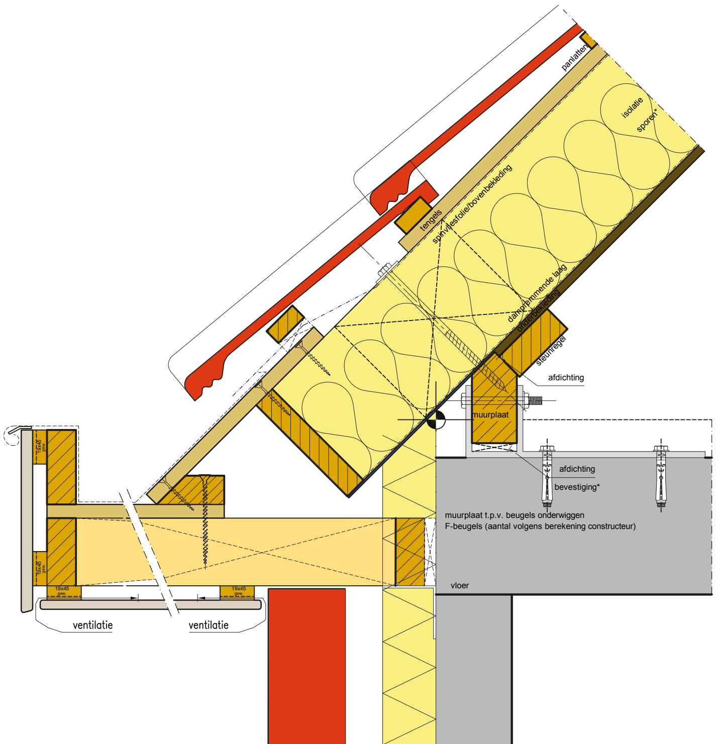
Detail 17: dakgootconstructie
