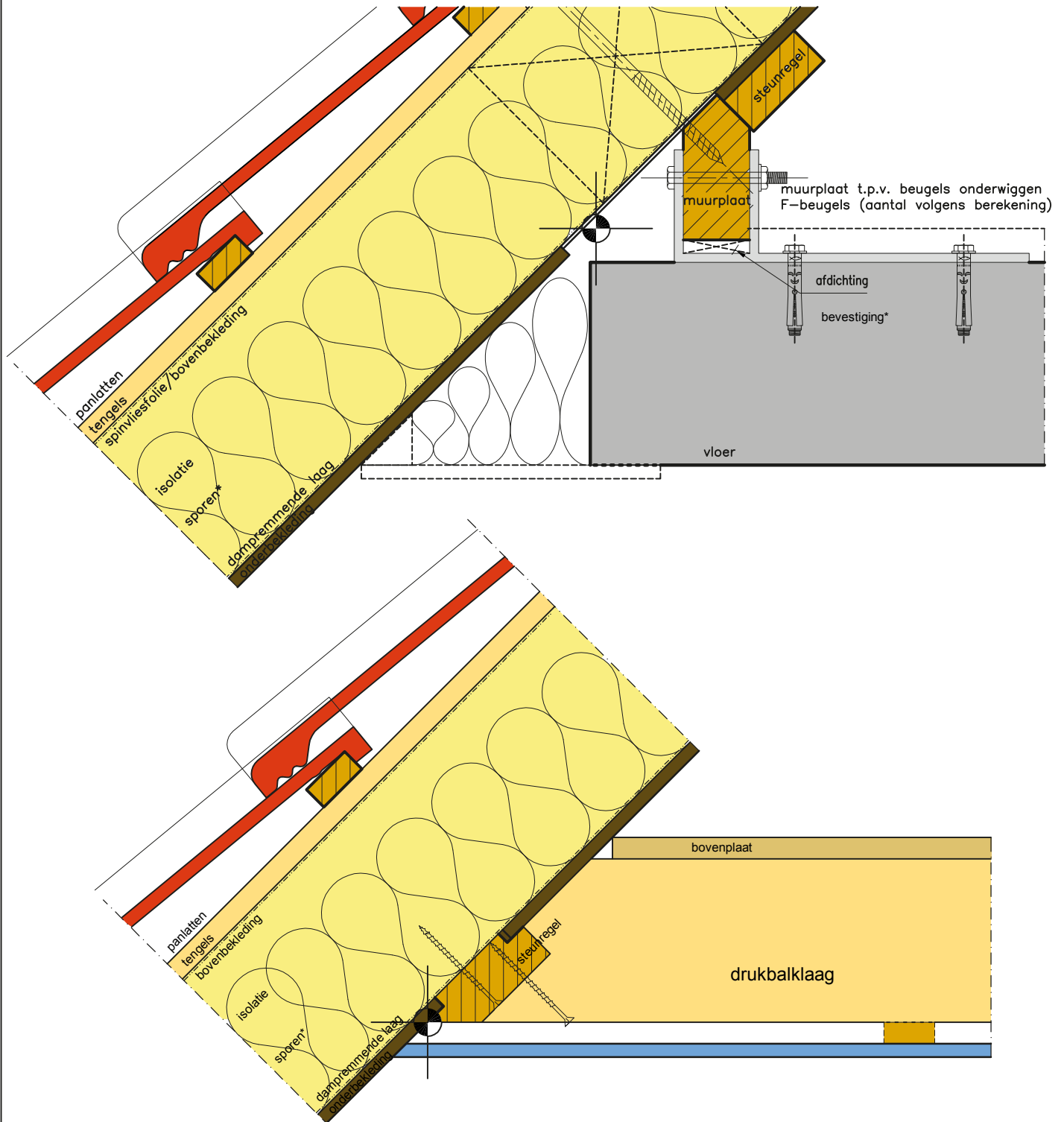
Detail 11: aansluiting vloer-dakconstructie
