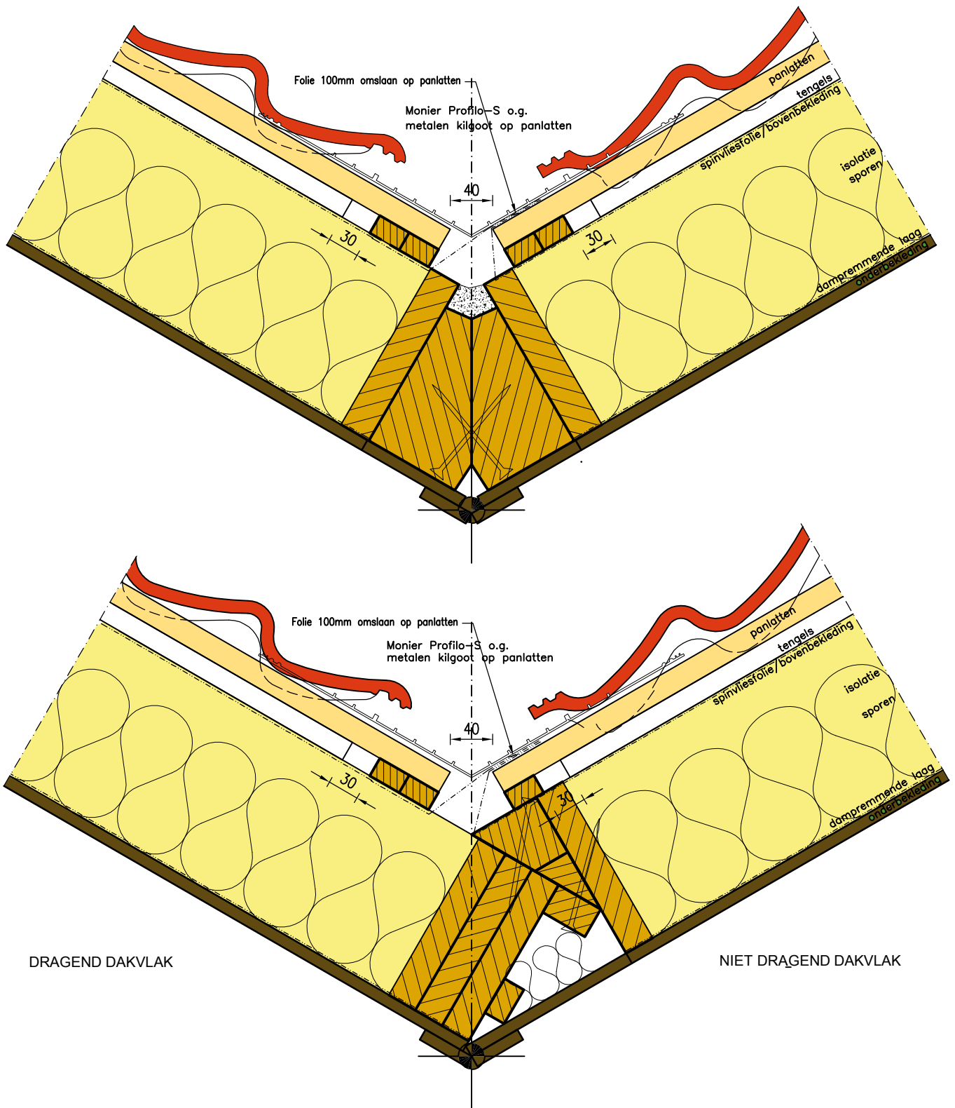
Detail 20a: kilkeperconstructie met kilgoot op panlatten
