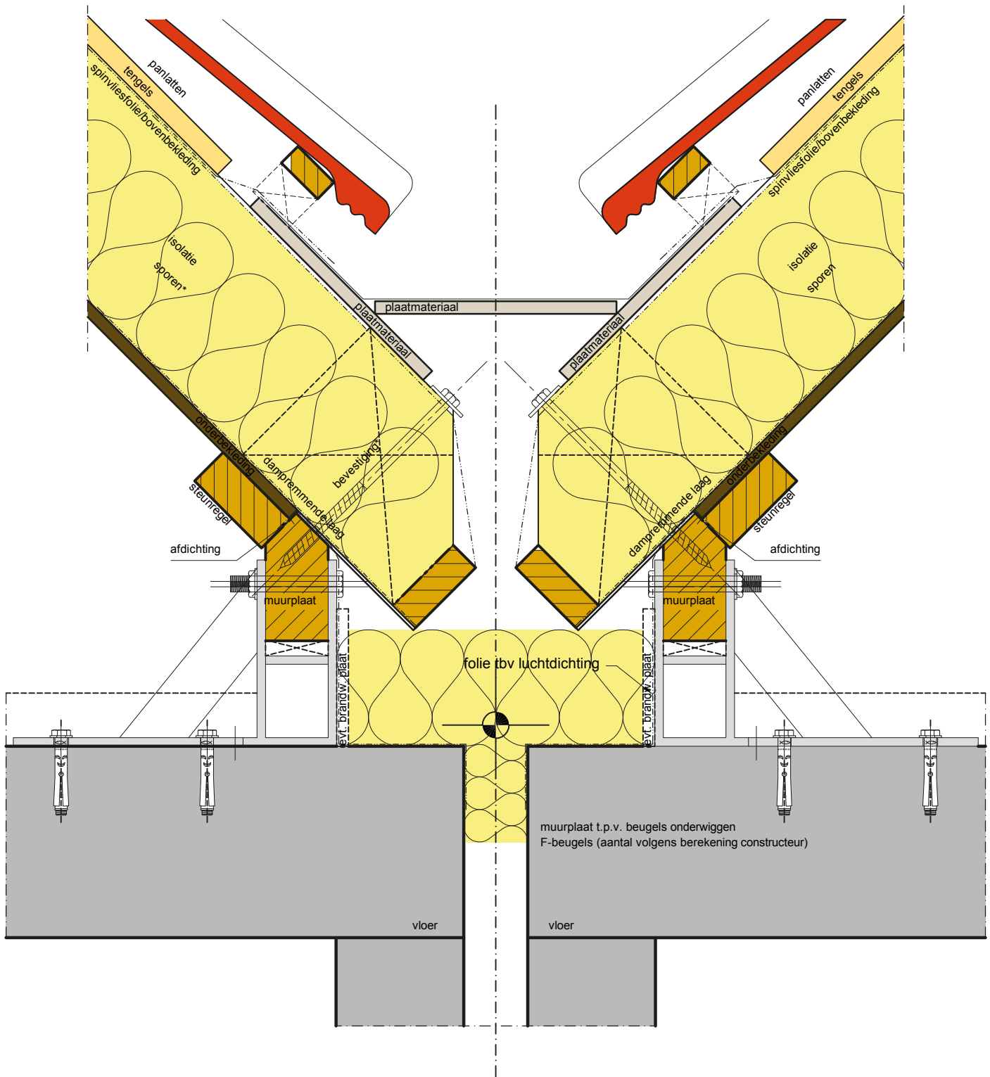
Detail 5: woningscheidende zakgootconstructie
